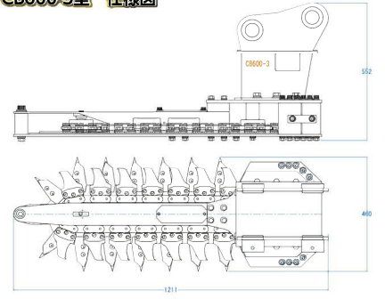
CB600-3型 仕様図
