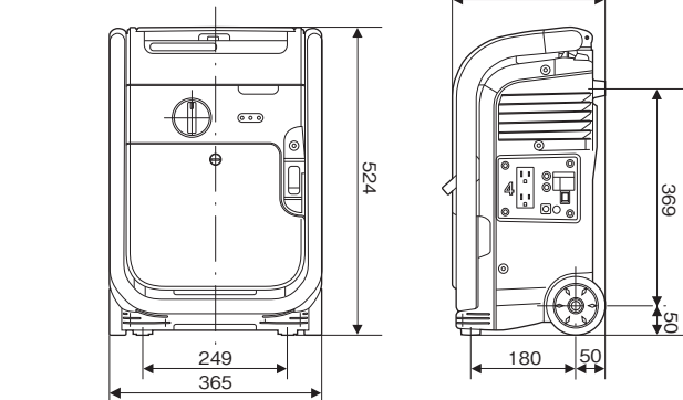
外観寸法図
