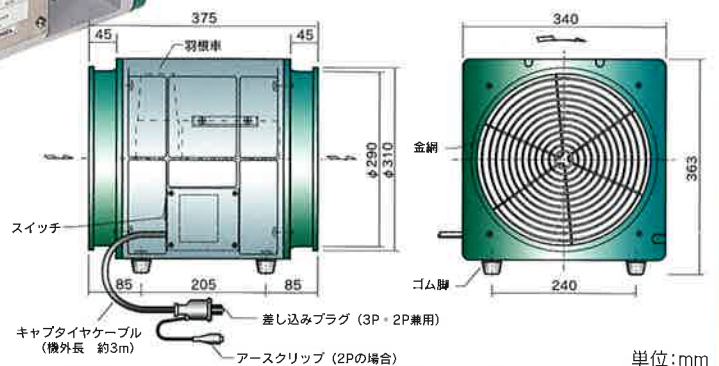
■外形寸法図
